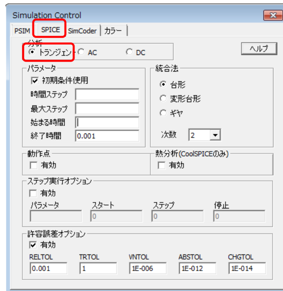
図 2-4 過渡解析の詳細設定画面
