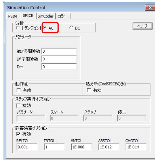
図 2-5 AC 解析パラメータ設定画面
