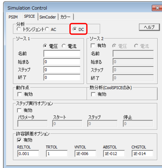
図 2-6 DC 解析パラメータ設定画面
